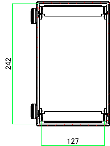
B-B ( 1 : 4.5 )
