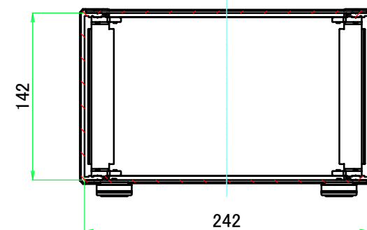
A-A ( 1 : 4.5 )
