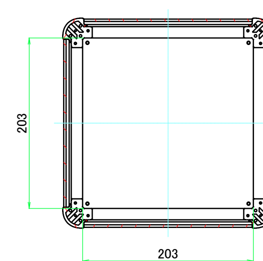
C-C ( 1 : 4.5 )
